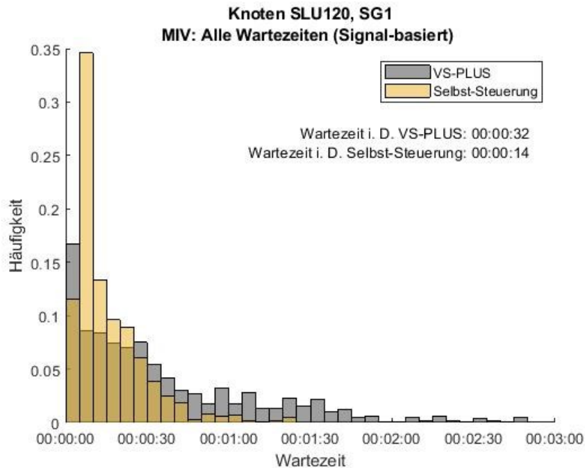
Abbildung 140: Häufigkeitsverteilung der Wartezeiten für den MIV in der dienstags Morgenspitze, Signalgeber 1, Knoten SLU120. In Grau ist die Verteilung des Nullfalles (VS-PLUS) und in Gelb die der Selbst-Steuerung abgebildet.
