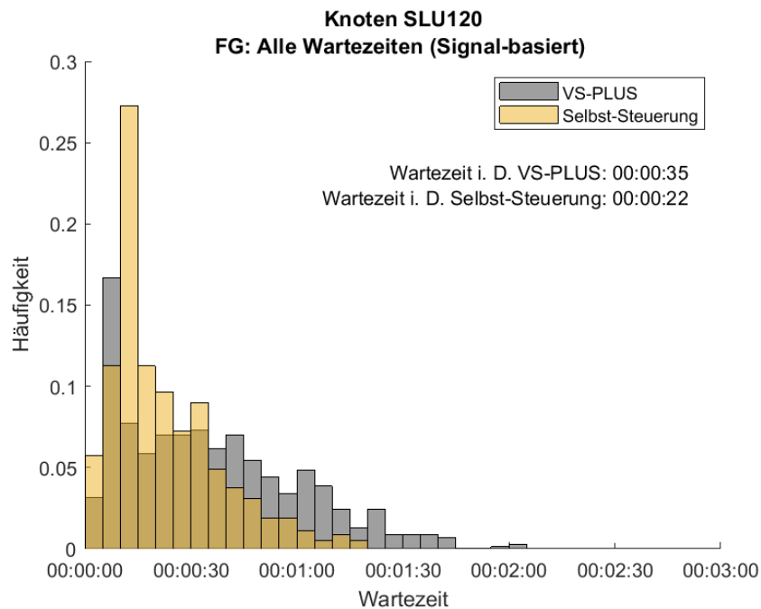
Abbildung 18: Häufigkeitsverteilung der Wartezeiten für den FV am Dienstag, Knoten SLU120. In Grau ist die Verteilung des Nullfalles (VS-PLUS) und in Gelb die der Selbst-Steuerung abgebildet.
