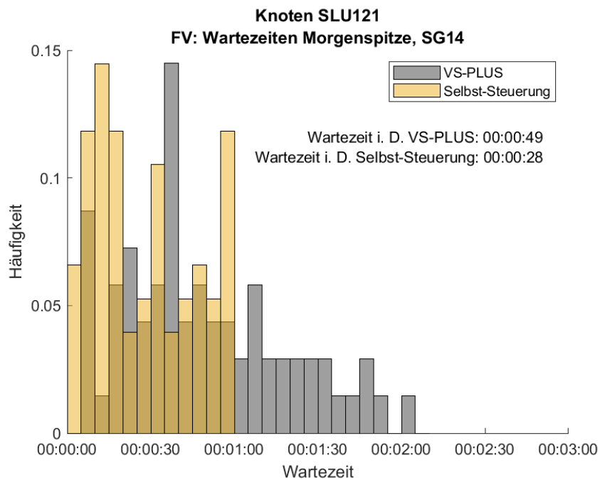
Abbildung 96: Häufigkeitsverteilung der Wartezeiten für den FV am Signalgeber 14 in der Abendspitze am Knoten SLU121. In Grau ist die Verteilung des Nullfalles (VS-PLUS) und in Gelb die der Selbst-Steuerung abgebildet.
