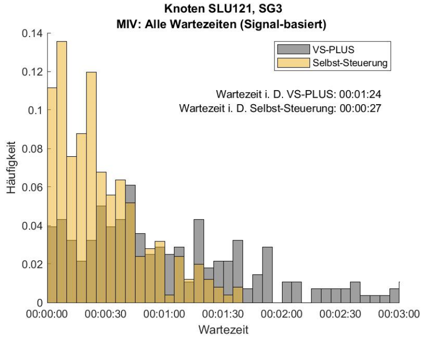
Abbildung 153: Häufigkeitsverteilung der Wartezeiten für den MIV in der dienstags Morgenspitze, Signalgeber 3, Knoten SLU121. In Grau ist die Verteilung des Nullfalles (VS-PLUS) und in Gelb die der Selbst-Steuerung abgebildet.
