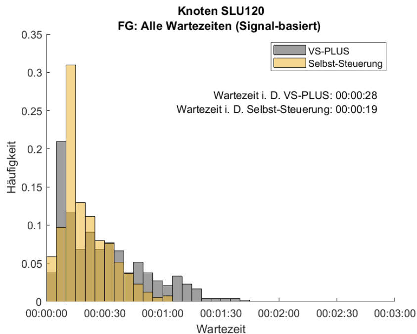
Abbildung 19: Häufigkeitsverteilung der Wartezeiten für den FV am Samstag, Knoten SLU120. In Grau ist die Verteilung des Nullfalles (VS-PLUS) und in Gelb die der Selbst-Steuerung abgebildet.
