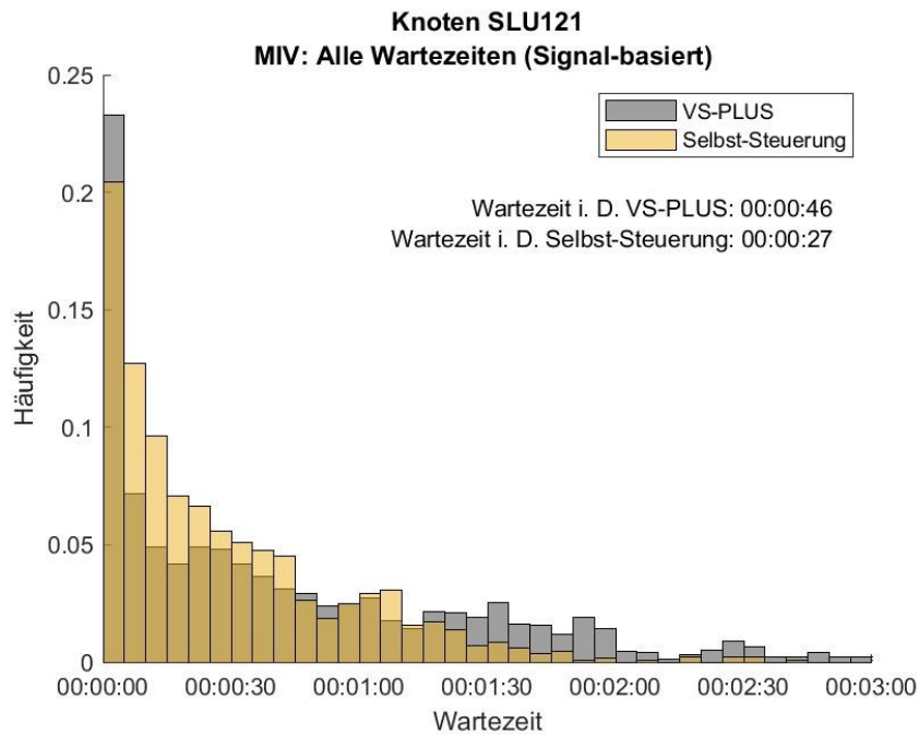
Abbildung 58: Häufigkeitsverteilung der Wartezeiten für den MIV in der dienstags Morgenspitze, Knoten SLU121. In Grau ist die Verteilung des Nullfalles (VS-PLUS) und in Gelb die der Selbst-Steuerung abgebildet.
