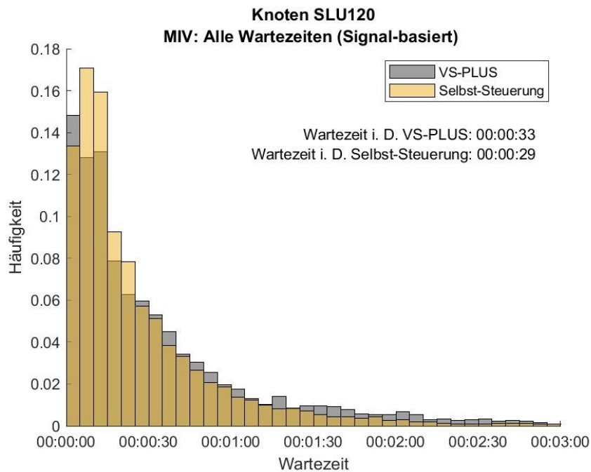
Abbildung 138: Häufigkeitsverteilung der Wartezeiten für den MIV am Donnerstag, Knoten SLU120. In Grau ist die Verteilung des Nullfalles (VS-PLUS) und in Gelb die der Selbst-Steuerung abgebildet.
