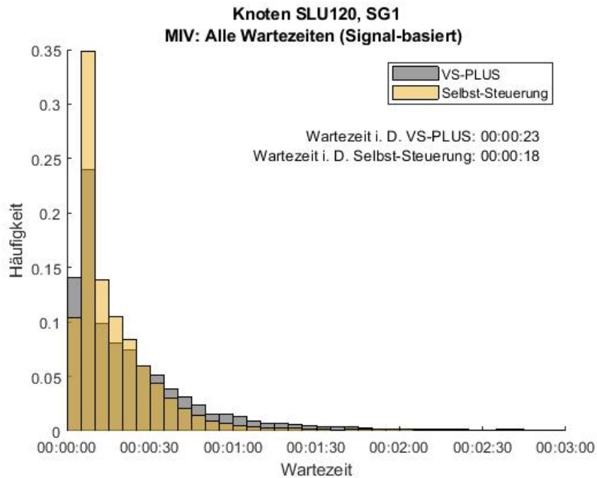
Abbildung 148: Häufigkeitsverteilung der Wartezeiten für den MIV, Signalgeber 1, Knoten SLU120. In Grau ist die Verteilung des Nullfalles (VS-PLUS) und in Gelb die der Selbst-Steuerung abgebildet.
