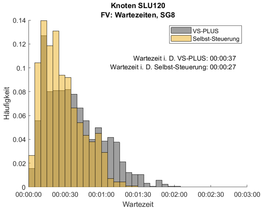
Abbildung 80: Häufigkeitsverteilung der Wartezeiten für den FV am Signalgeber 8 im gesamten Messzeitraum am Knoten SLU120. In Grau ist die Verteilung des Nullfalles (VS-PLUS) und in Gelb die der Selbst-Steuerung abgebildet.
