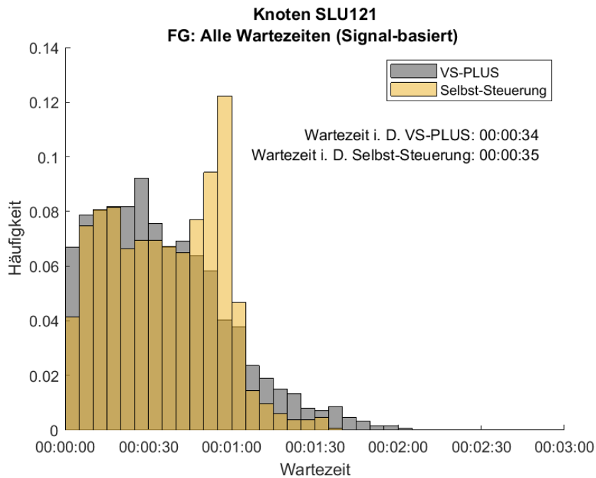
Abbildung 86: Häufigkeitsverteilung der Wartezeiten für den FV, freitags am Knoten SLU121. In Grau ist die Verteilung des Nullfalles (VS-PLUS) und in Gelb die der Selbst-Steuerung abgebildet.
