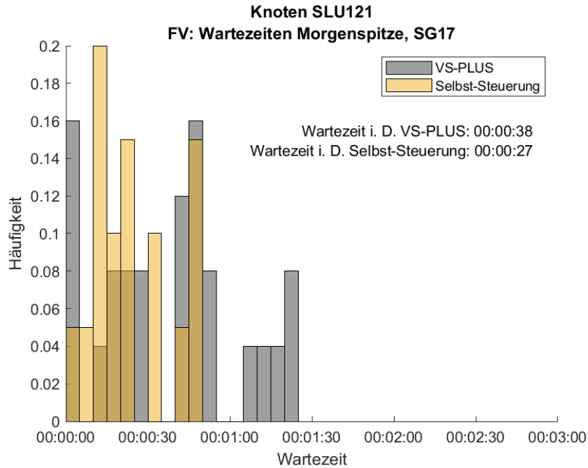
Abbildung g1: Häufigkeitsverteilung der Wartezeiten für den FV am Signalgeber 17 in der Morgenspitze am Knoten SLU121. In Grau ist die Verteilung des Nullfalles (VS-PLUS) und in Gelb die der Selbst-Steuerung abgebildet.
