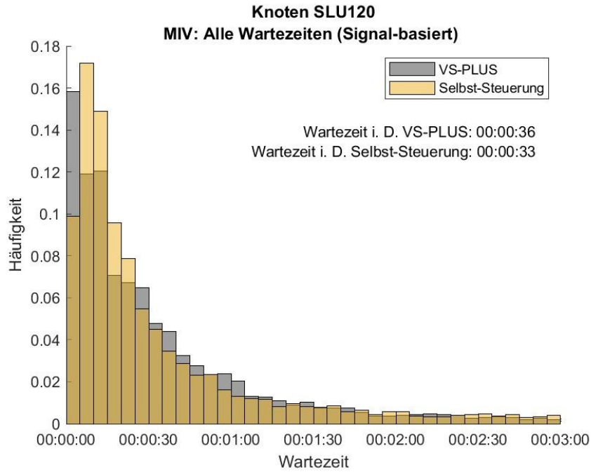
Abbildung 137: Häufigkeitsverteilung der Wartezeiten für den MIV am Mittwoch, Knoten SLU120. In Grau ist die Verteilung des Nullfalles (VS-PLUS) und in Gelb die der Selbst-Steuerung abgebildet.
