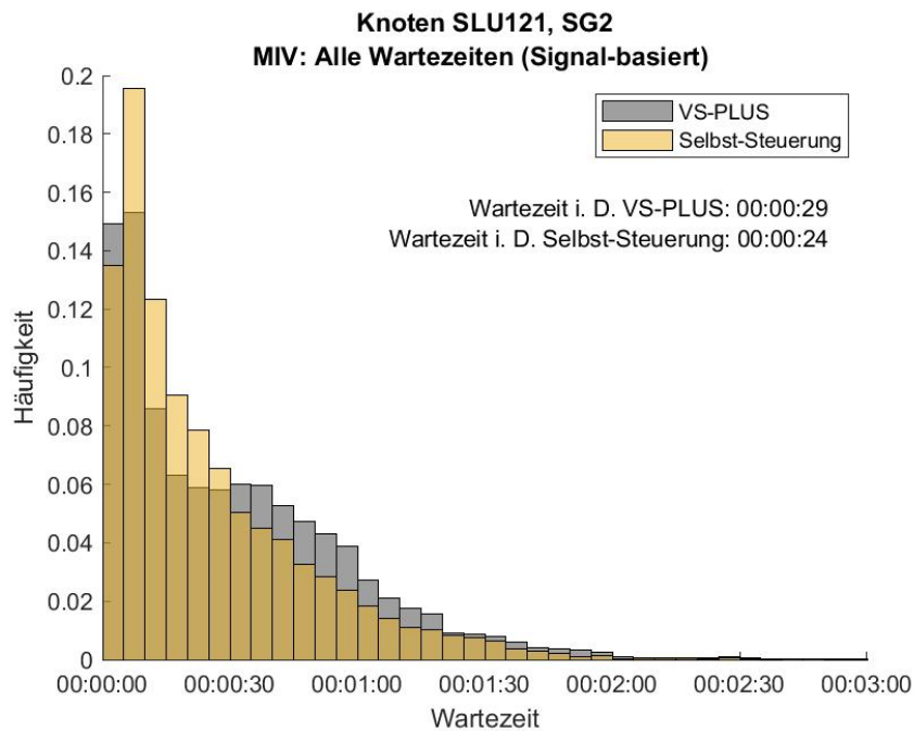
Abbildung 160: Häufigkeitsverteilung der Wartezeiten für den MIV im gesamten Messzeitraum, Signalgeber 2, Knoten SLU121. In Grau ist die Verteilung des Nullfalles (VS-PLUS) und in Gelb die der Selbst-Steuerung abgebildet.
