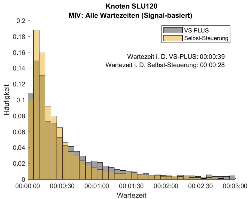
Abbildung 46: Häufigkeitsverteilung der Wartezeiten für den MIV am Dienstag, Knoten SLU120. In Grau ist die Verteilung des Nullfalles (VS-PLUS) und in Gelb die der Selbst-Steuerung abgebildet.
