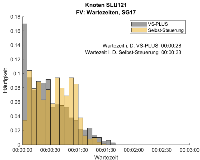
Abbildung 102: Häufigkeitsverteilung der Wartezeiten für den FV am Signalgeber 17 im gesamten Messzeitraum am Knoten SLU121. In Grau ist die Verteilung des Nullfalles (VS-PLUS) und in Gelb die der Selbst-Steuerung abgebildet.
