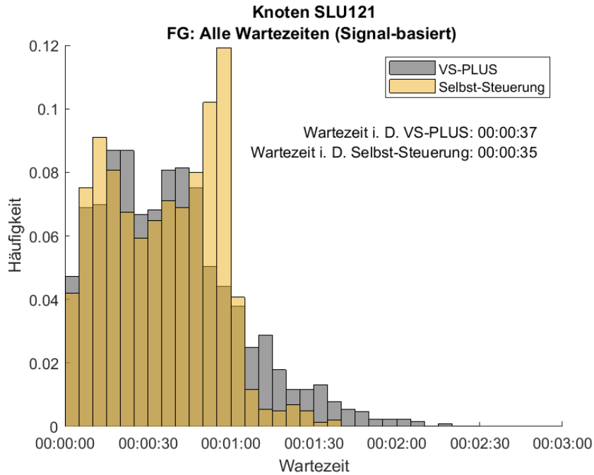
Abbildung 85: Häufigkeitsverteilung der Wartezeiten für den FV, donnerstags am Knoten SLU121. In Grau ist die Verteilung des Nullfalles (VS-PLUS) und in Gelb die der Selbst-Steuerung abgebildet.
