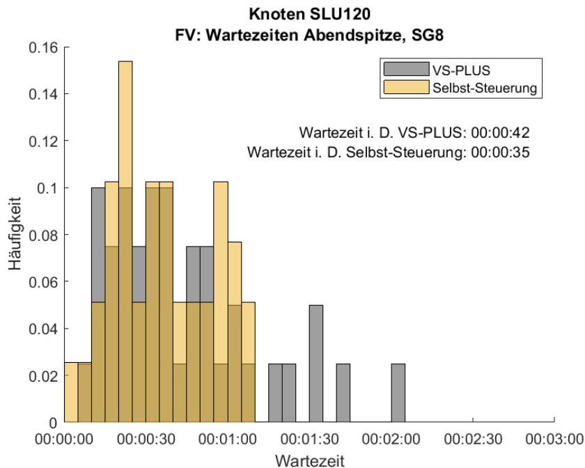
Abbildung 76: Häufigkeitsverteilung der Wartezeiten für den FV am Signalgeber 8 in der Abendspitze am Knoten SLU120. In Grau ist die Verteilung des Nullfalles (VS-PLUS) und in Gelb die der Selbst-Steuerung abgebildet.
