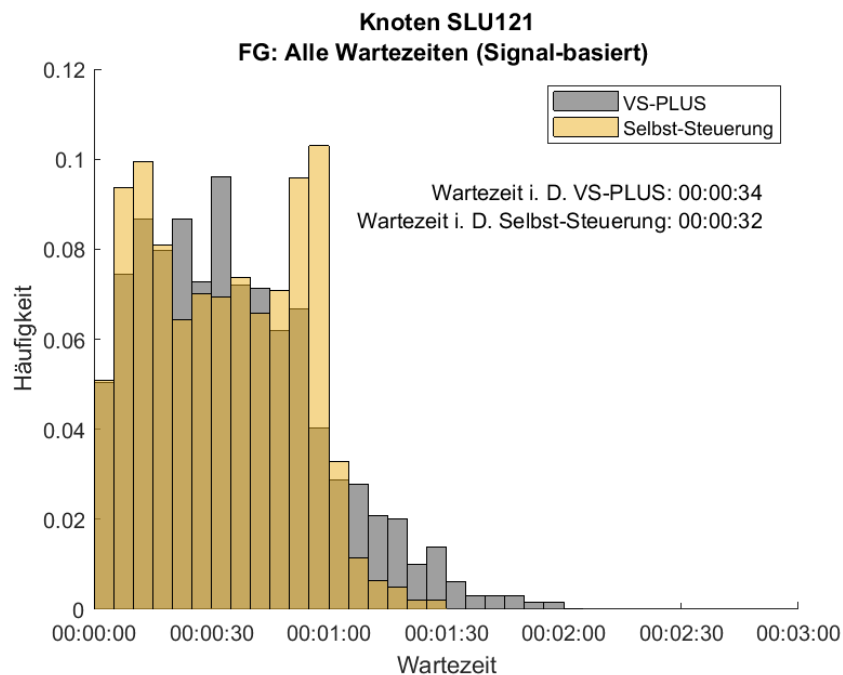
Abbildung 24: Häufigkeitsverteilung der Wartezeiten für den FV am Montag, Knoten SLU121. In Grau ist die Verteilung des Nullfalles (VS-PLUS) und in Gelb die der Selbst-Steuerung abgebildet.
