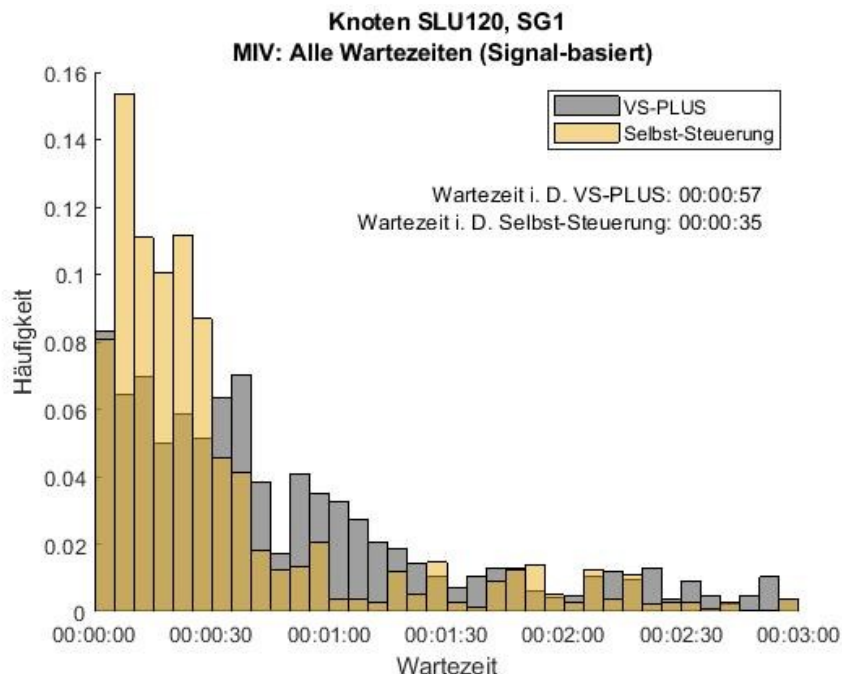
Abbildung 144: Häufigkeitsverteilung der Wartezeiten für den MIV in der dienstags Abendspitze, Signalgeber 1, Knoten SLU120. In Grau ist die Verteilung des Nullfalles (VS-PLUS) und in Gelb die der Selbst-Steuerung abgebildet.
