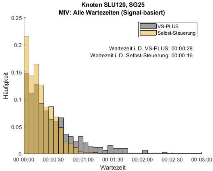
Abbildung 147: Häufigkeitsverteilung der Wartezeiten für den MIV in der dienstags Abendspitze, Signalgeber 25, Knoten SLU120. In Grau ist die Verteilung des Nullfalles (VS-PLUS) und in Gelb die der Selbst-Steuerung abgebildet.
