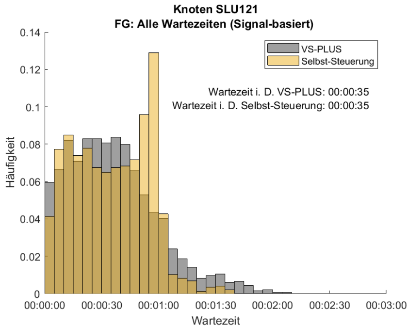
Abbildung 84: Häufigkeitsverteilung der Wartezeiten für den FV, mittwochs am Knoten SLU121. In Grau ist die Verteilung des Nullfalles (VS-PLUS) und in Gelb die der Selbst-Steuerung abgebildet.
