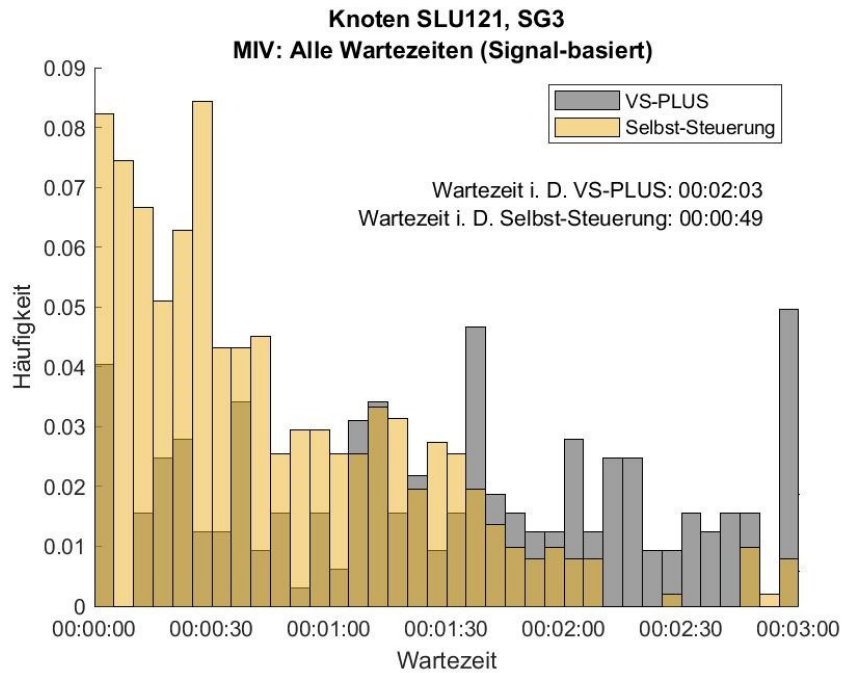
Abbildung 157: Häufigkeitsverteilung der Wartezeiten für den MIV in der dienstags Abendspitze, Signalgeber 3, Knoten SLU121. In Grau ist die Verteilung des Nullfalles (VS-PLUS) und in Gelb die der Selbst-Steuerung abgebildet.
