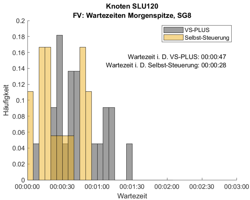
Abbildung 72: Häufigkeitsverteilung der Wartezeiten für den FV am Signalgeber 8 in der Morgenspitze am Knoten SLU120. In Grau ist die Verteilung des Nullfalles (VS-PLUS) und in Gelb die der Selbst-Steuerung abgebildet.
