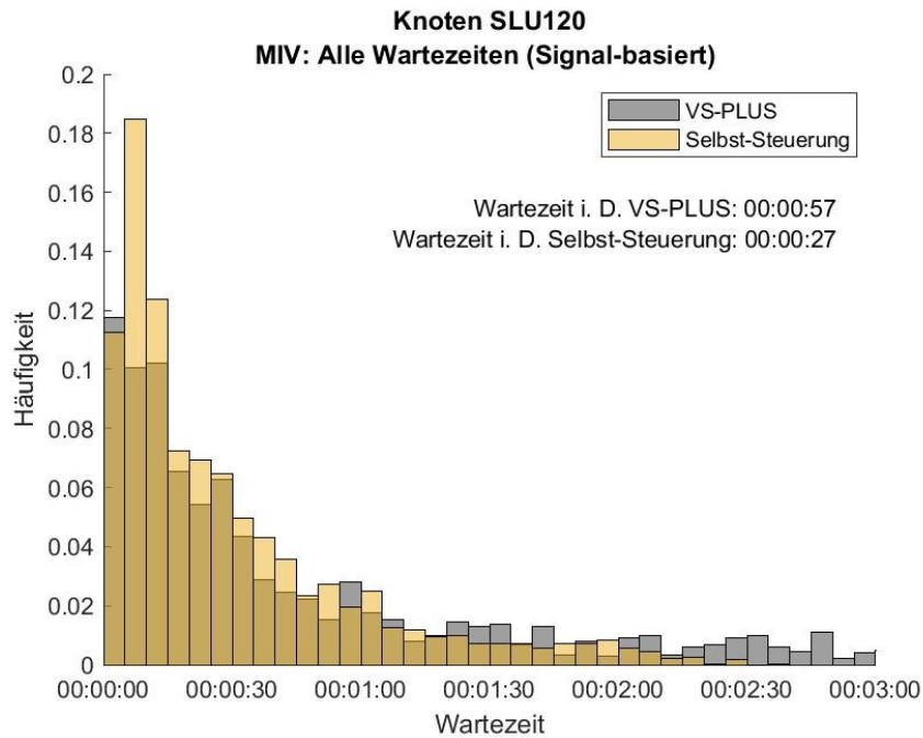
Abbildung 48: Häufigkeitsverteilung der Wartezeiten für den MIV in der dienstags Morgenspitze, Knoten SLU120. In Grau ist die Verteilung des Nullfalles (VS-PLUS) und in Gelb die der Selbst-Steuerung abgebildet.
