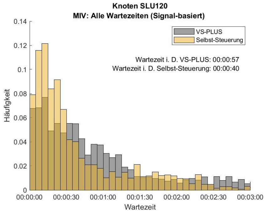
Abbildung 50: Häufigkeitsverteilung der Wartezeiten für den MIV in der dienstags Abendspitze, Knoten SLU120. In Grau ist die Verteilung des Nullfalles (VS-PLUS) und in Gelb die der Selbst-Steuerung abgebildet.
