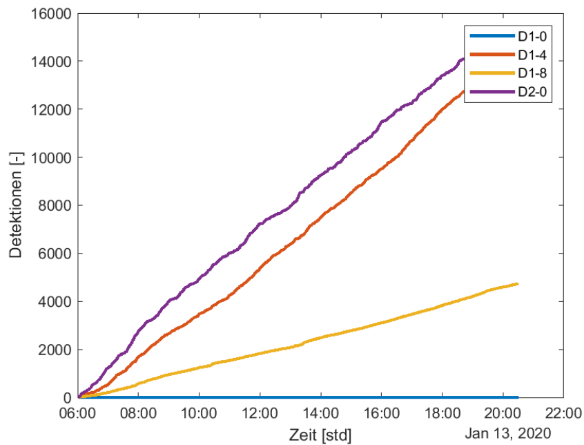
Abbildung 11: Kumulierte Detektorbelegungen am Knoten SLU121 für D 1-o, D 1-4, D 1-8, D 2-o.
