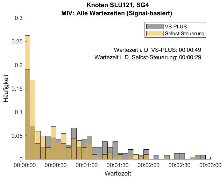
Abbildung 154: Häufigkeitsverteilung der Wartezeiten für den MIV in der dienstags Morgenspitze, Signalgeber 4, Knoten SLU121. In Grau ist die Verteilung des Nullfalles (VS-PLUS) und in Gelb die der Selbst-Steuerung abgebildet.
