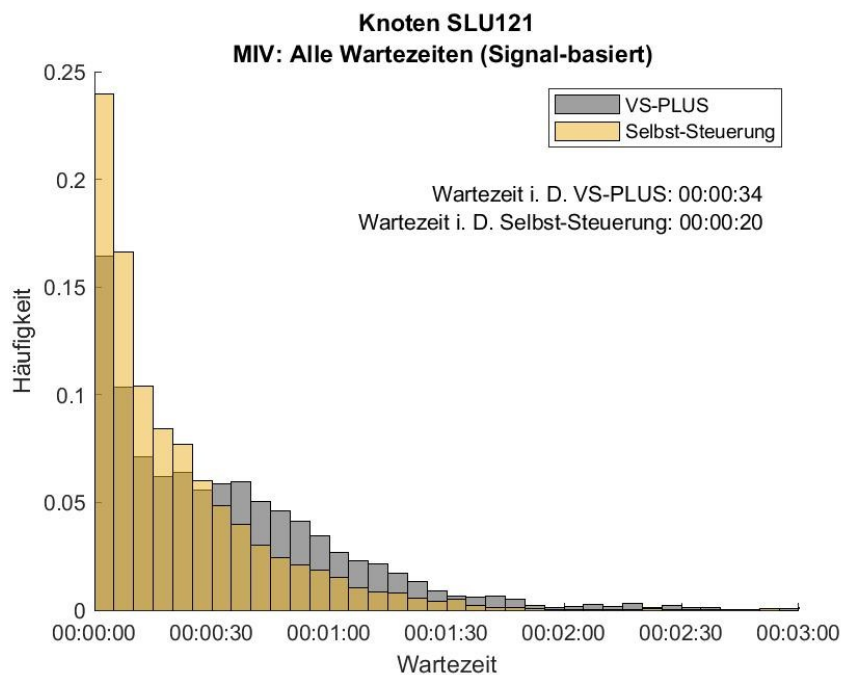
Abbildung 55: Häufigkeitsverteilung der Wartezeiten für den MIV am Montag, Knoten SLU121. In Grau ist die Verteilung des Nullfalles (VS-PLUS) und in Gelb die der Selbst-Steuerung abgebildet.
