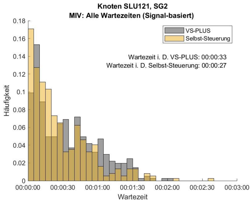
Abbildung 156: Häufigkeitsverteilung der Wartezeiten für den MIV in der dienstags Abendspitze, Signalgeber 2, Knoten SLU121. In Grau ist die Verteilung des Nullfalles (VS-PLUS) und in Gelb die der Selbst-Steuerung abgebildet.
