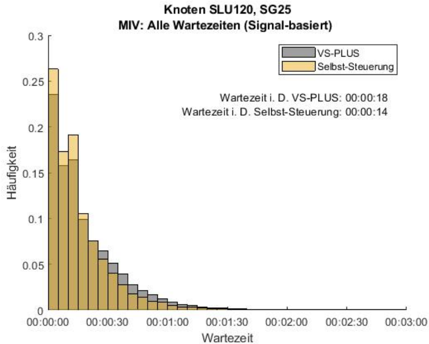
Abbildung 151: Häufigkeitsverteilung der Wartezeiten für den MIV, Signalgeber 25, Knoten SLU120. In Grau ist die Verteilung des Nullfalles (VS-PLUS) und in Gelb die der Selbst-Steuerung abgebildet.
