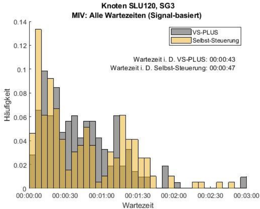
Abbildung 145: Häufigkeitsverteilung der Wartezeiten für den MIV in der dienstags Abendspitze, Signalgeber 3, Knoten SLU120. In Grau ist die Verteilung des Nullfalles (VS-PLUS) und in Gelb die der Selbst-Steuerung abgebildet.
