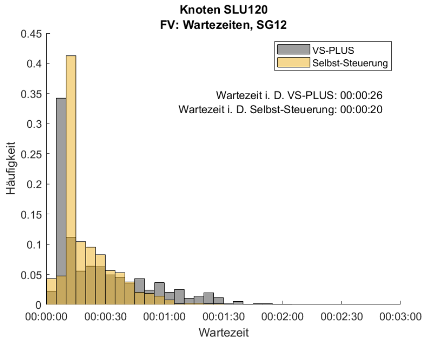
Abbildung 82: Häufigkeitsverteilung der Wartezeiten für den FV am Signalgeber 12 im gesamten Messzeitraum am Knoten SLU120. In Grau ist die Verteilung des Nullfalles (VS-PLUS) und in Gelb die der Selbst-Steuerung abgebildet.
