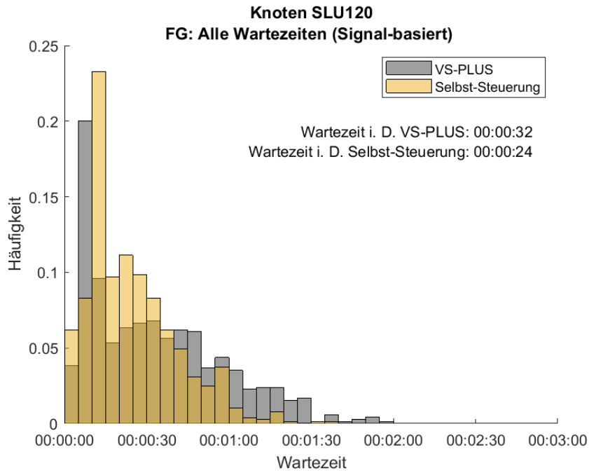
Abbildung 71: Häufigkeitsverteilung der Wartezeiten für den FV, freitags am Knoten SLU120. In Grau ist die Verteilung des Nullfalles (VS-PLUS) und in Gelb die der Selbst-Steuerung abgebildet.
