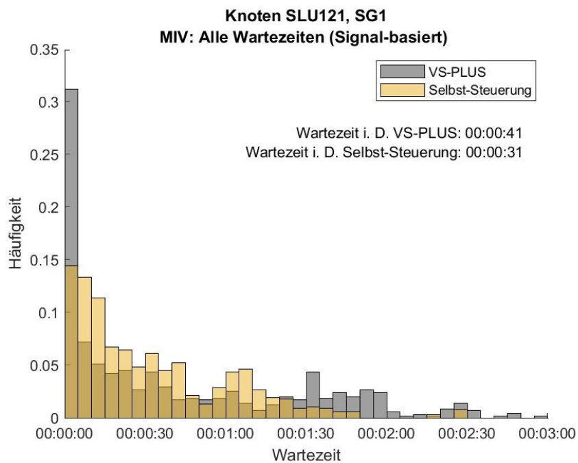
Abbildung 152: Häufigkeitsverteilung der Wartezeiten für den MIV in der dienstags Morgenspitze, Signalgeber 2, Knoten SLU121. In Grau ist die Verteilung des Nullfalles (VS-PLUS) und in Gelb die der Selbst-Steuerung abgebildet.
