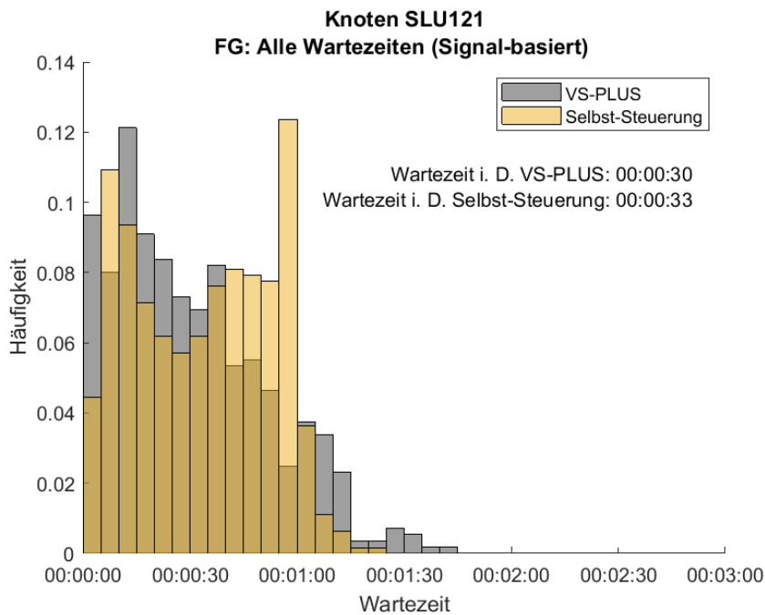
Abbildung 25: Häufigkeitsverteilung der Wartezeiten für den FV am Dienstag, Knoten SLU121. In Grau ist die Verteilung des Nullfalles (VS-PLUS) und in Gelb die der Selbst-Steuerung abgebildet.
