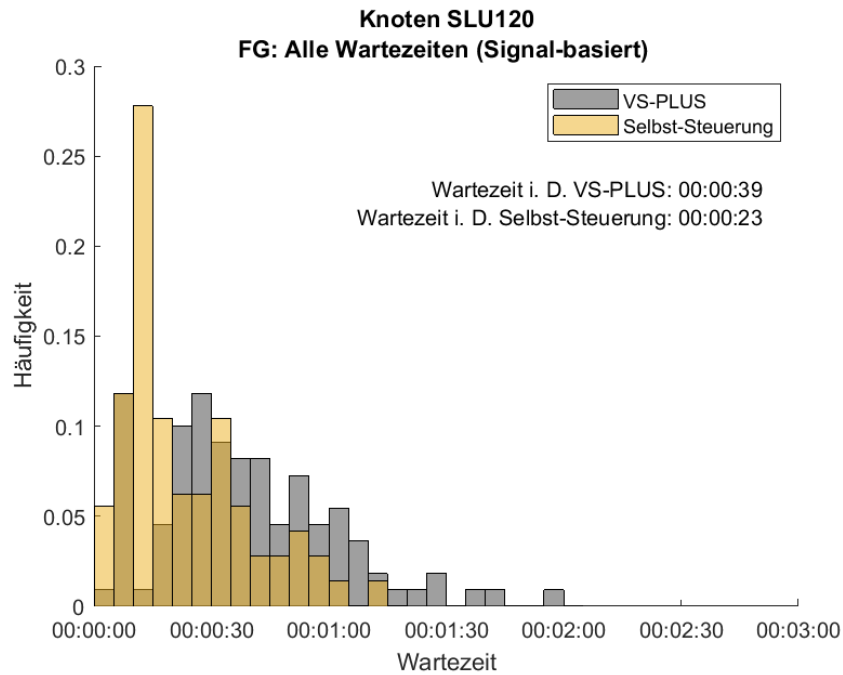
Abbildung 20: Häufigkeitsverteilung der Wartezeiten für den FV der Morgenspitze am Dienstag, Knoten SLU120. In Grau ist die Verteilung des Nullfalles (VS-PLUS) und in Gelb die der Selbst-Steuerung abgebildet.
