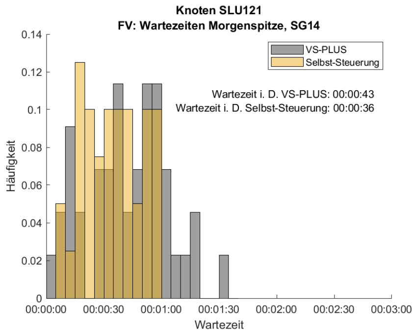
Abbildung 90: Häufigkeitsverteilung der Wartezeiten für den FV am Signalgeber 14 in der Morgenspitze am Knoten SLU121. In Grau ist die Verteilung des Nullfalles (VS-PLUS) und in Gelb die der Selbst-Steuerung abgebildet.
