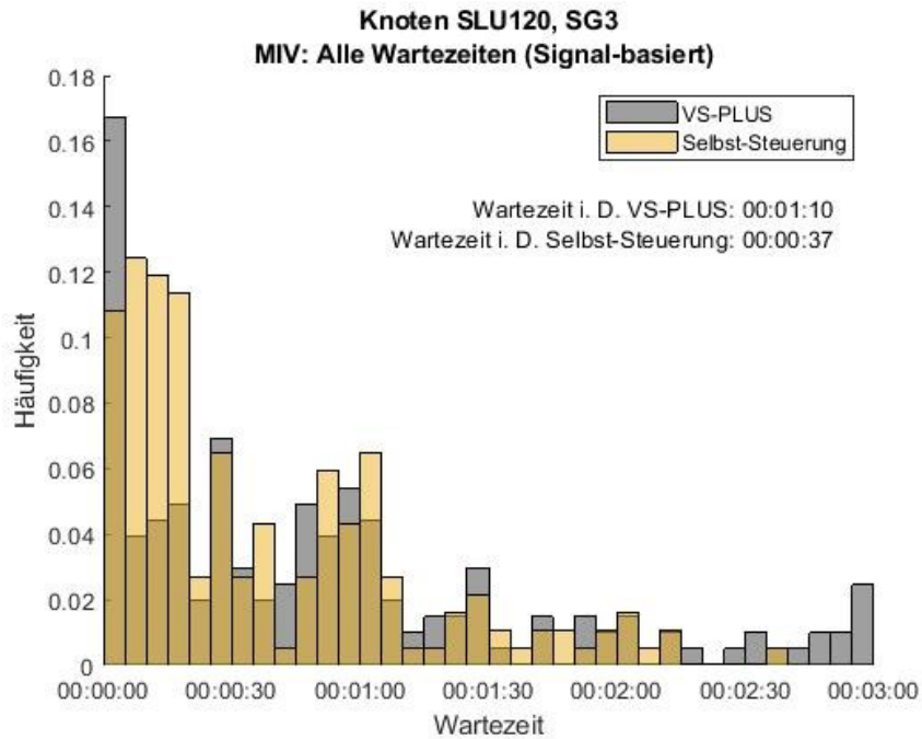
Abbildung 141: : Häufigkeitsverteilung der Wartezeiten für den MIV in der dienstags Morgenspitze, Signalgeber 3, Knoten SLU120. In Grau ist die Verteilung des Nullfalles (VS-PLUS) und in Gelb die der Selbst-Steuerung abgebildet.
