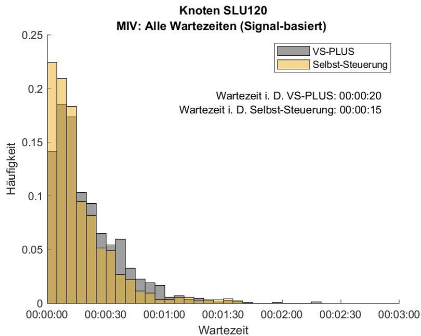
Abbildung 49: Häufigkeitsverteilung der Wartezeiten für den MIV im Mittagsverkehr des Dienstages, Knoten SLU120. In Grau ist die Verteilung des Nullfalles (VS-PLUS) und in Gelb die der Selbst-Steuerung abgebildet.
