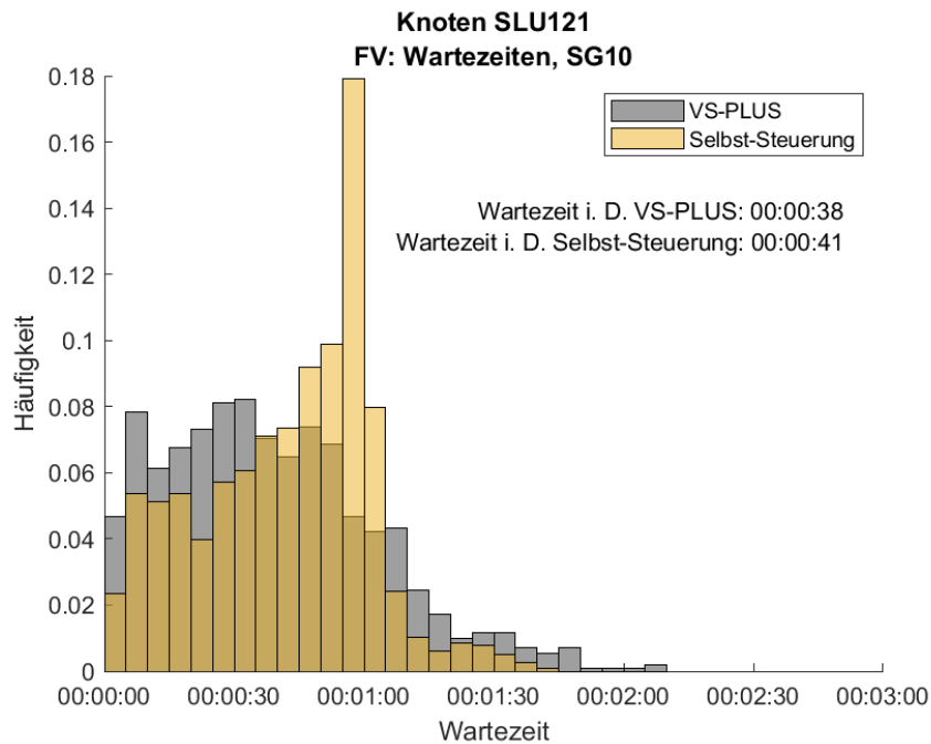
Abbildung 100: Häufigkeitsverteilung der Wartezeiten für den FV am Signalgeber 10 im gesamten Messzeitraum am Knoten SLU121. In Grau ist die Verteilung des Nullfalles (VS-PLUS) und in Gelb die der Selbst-Steuerung abgebildet.
