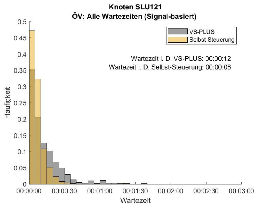
Abbildung 38: Häufigkeitsverteilung der Wartezeiten für den ÖV am Montag, Knoten SLU121. In Grau ist die Verteilung des Nullfalles (VS-PLUS) und in Gelb die der Selbst-Steuerung abgebildet.
