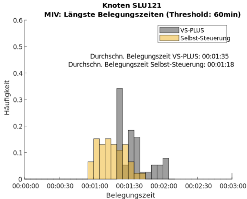
Abbildung 64: Belegungszeiten der Voranmeldedetektoren am Knoten SLU121 aggregiert auf eine Stunde Messzeitraum. In Grau ist die Verteilung des Nullfalles (VS-PLUS) und in Gelb die der Selbst-Steuerung abgebildet.
