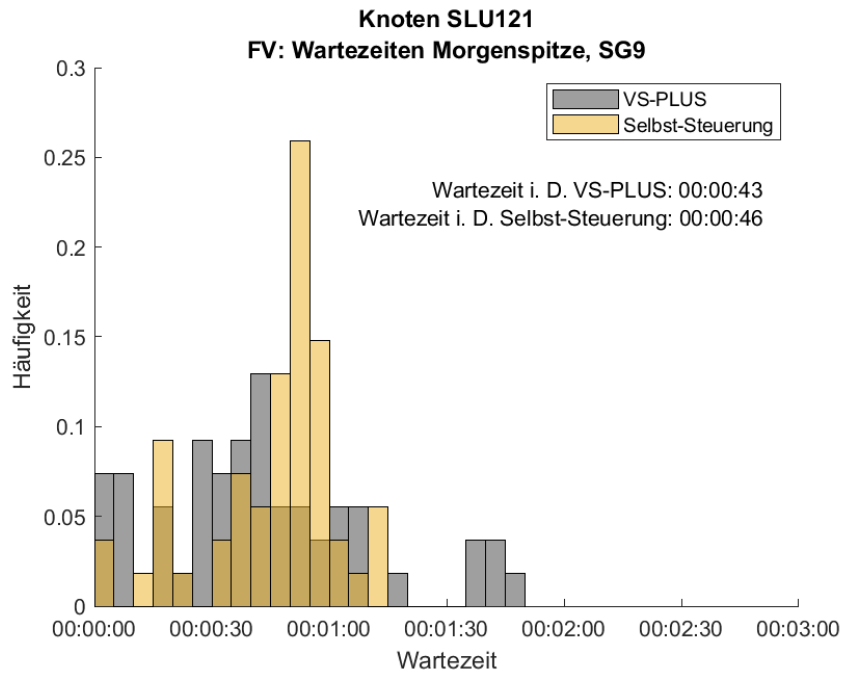
Abbildung 87: Häufigkeitsverteilung der Wartezeiten für den FV am Signalgeber 9 in der Morgenspitze am Knoten SLU121. In Grau ist die Verteilung des Nullfalles (VS-PLUS) und in Gelb die der Selbst-Steuerung abgebildet.
