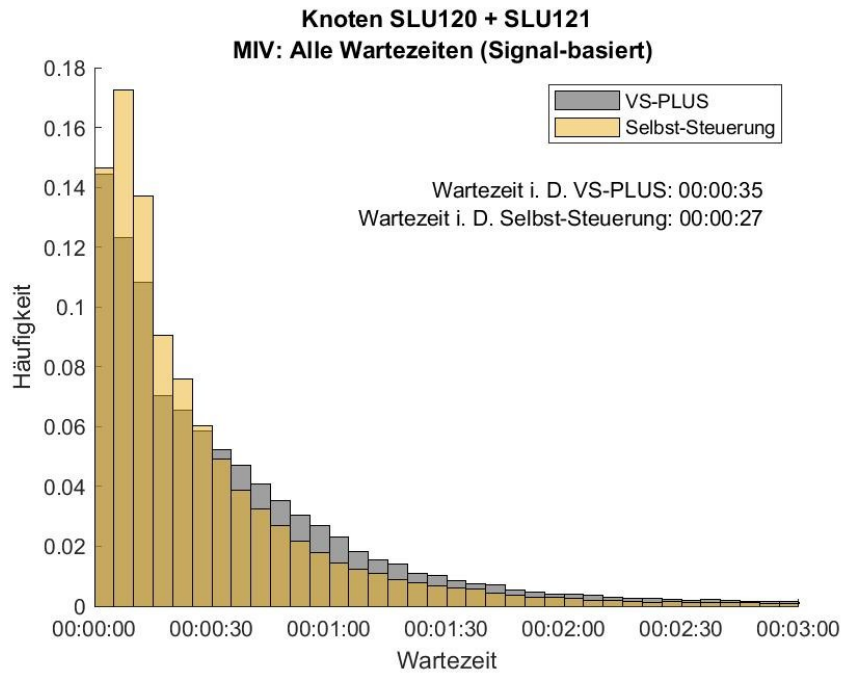
Abbildung 67: Aggregierte Wartezeiten für den MIV am Knoten SLU120 und SLU121 über den gesamten Messzeitraum. In Grau ist die Verteilung des Nullfalles (VS-PLUS) und in Gelb die der Selbst-Steuerung abgebildet.
