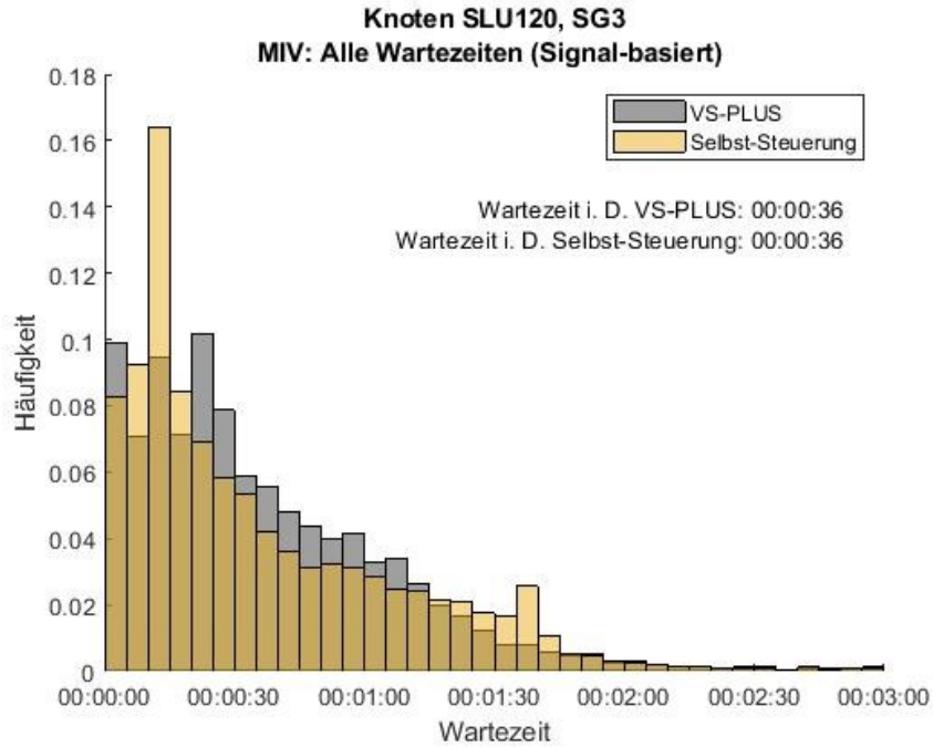
Abbildung 149: Häufigkeitsverteilung der Wartezeiten für den MIV, Signalgeber 3, Knoten SLU120. In Grau ist die Verteilung des Nullfalles (VS-PLUS) und in Gelb die der Selbst-Steuerung abgebildet.
