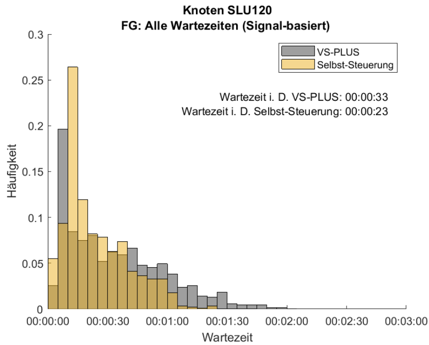
Abbildung 69: Häufigkeitsverteilung der Wartezeiten für den FV, mittwochs am Knoten SLU120. In Grau ist die Verteilung des Nullfalles (VS-PLUS) und in Gelb die der Selbst-Steuerung abgebildet.
