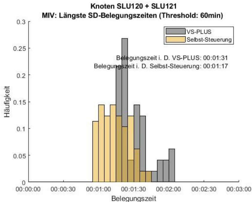
Abbildung 68: Längste Belegungszeiten (Grenzwert 60 Minuten) für das gesamte Untersuchungsgebiet.
