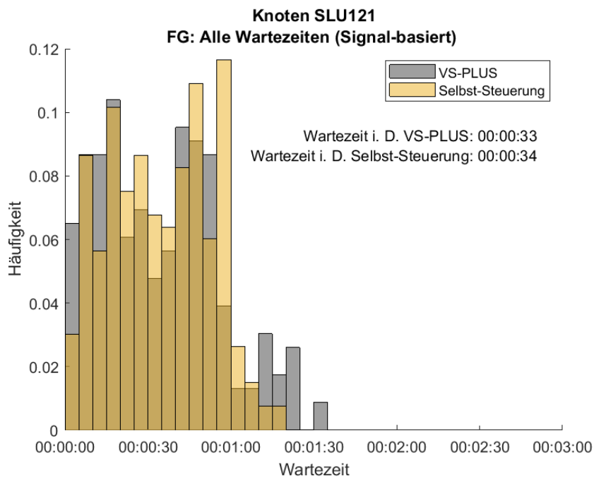
Abbildung 29: Häufigkeitsverteilung der Wartezeiten für den FV in der dienstags Abendspitze, Knoten SLU121. In Grau ist die Verteilung des Nullfalles (VS-PLUS) und in Gelb die der Selbst-Steuerung abgebildet.
