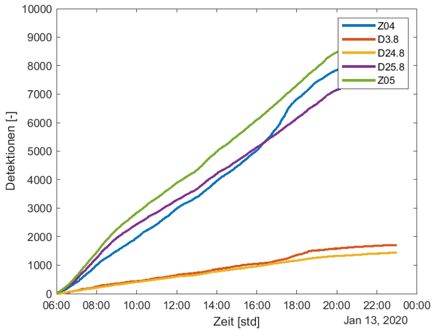
Abbildung 169: Kumulierte Detektionen für die Detektoren Z04, D3.8, D24.8, D25.8 und Z05 am Knoten SLU120.
