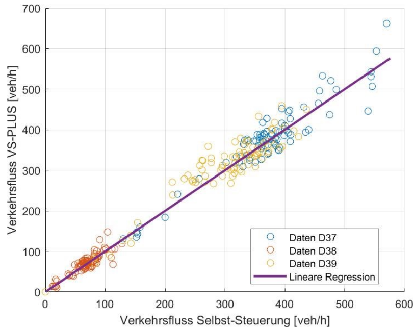
Abbildung 16: Gegenüberstellung der Verkehrsflüsse in [veh/h] der Zählschlaufen am SLU121. Die blauen, orangen und gelben Datenpunkte geben den Zusammenhang mit der korrespondierenden Regressionsgerade für D37, D38 und D39 an. Das Bestimmtheitsmass kann jeweils mit 0,99 angegeben werden. Die Regressionskoeffizienten \beta_1 sind mit 1,00 definiert.
