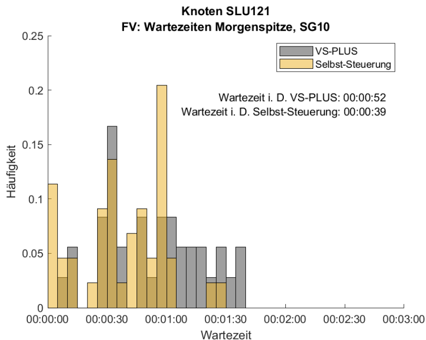
Abbildung 88: Häufigkeitsverteilung der Wartezeiten für den FV am Signalgeber 10 in der Morgenspitze am Knoten SLU121. In Grau ist die Verteilung des Nullfalles (VS-PLUS) und in Gelb die der Selbst-Steuerung abgebildet.
