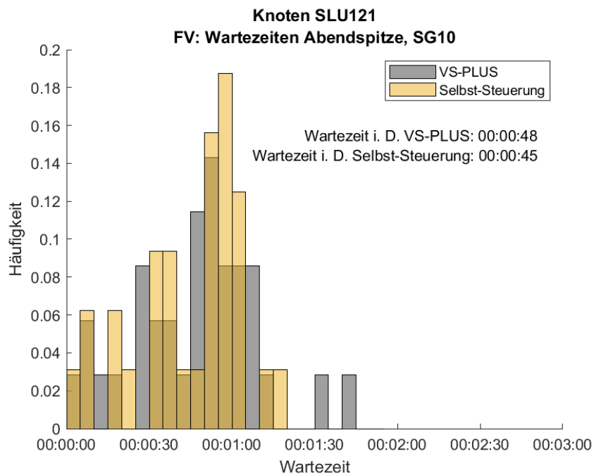
Abbildung 94: Häufigkeitsverteilung der Wartezeiten für den FV am Signalgeber 10 in der Abendspitze am Knoten SLU121. In Grau ist die Verteilung des Nullfalles (VS-PLUS) und in Gelb die der Selbst-Steuerung abgebildet.
