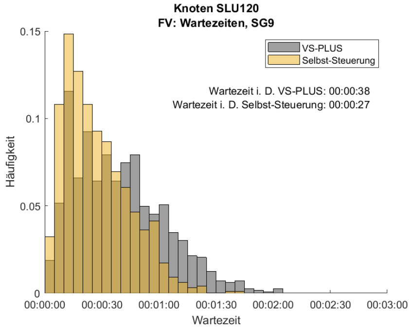
Abbildung 79: Häufigkeitsverteilung der Wartezeiten für den FV am Signalgeber 13 in der Abendspitze am Knoten SLU120. In Grau ist die Verteilung des Nullfalles (VS-PLUS) und in Gelb die der Selbst-Steuerung abgebildet.
