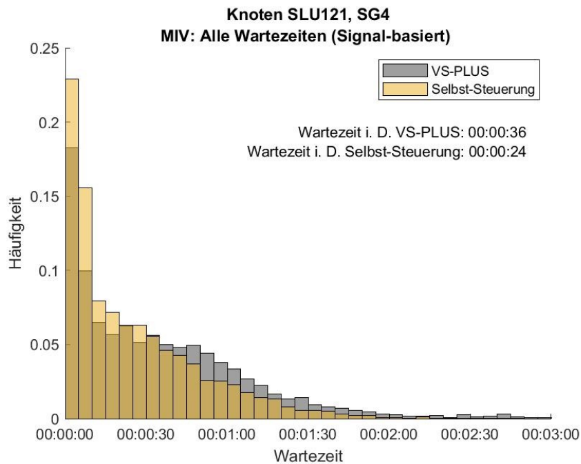
Abbildung 162: Häufigkeitsverteilung der Wartezeiten für den MIV im gesamten Messzeitraum, Signalgeber 4, Knoten SLU121. In Grau ist die Verteilung des Nullfalles (VS-PLUS) und in Gelb die der Selbst-Steuerung abgebildet.
