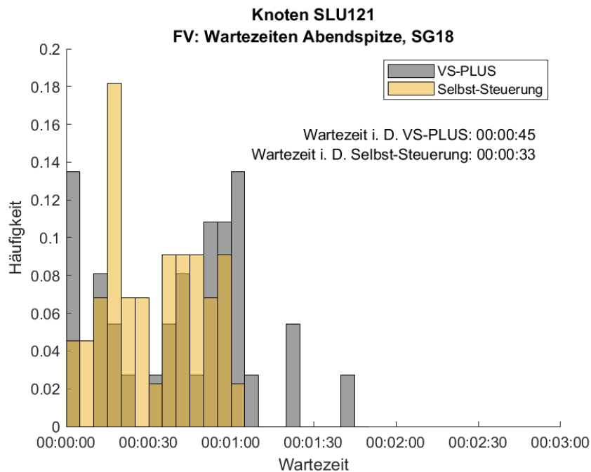
Abbildung 98: Häufigkeitsverteilung der Wartezeiten für den FV am Signalgeber 18 in der Abendspitze am Knoten SLU121. In Grau ist die Verteilung des Nullfalles (VS-PLUS) und in Gelb die der Selbst-Steuerung abgebildet.
