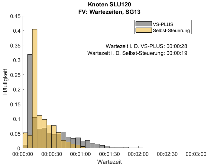
Abbildung 83: Häufigkeitsverteilung der Wartezeiten für den FV am Signalgeber 13 im gesamten Messzeitraum am Knoten SLU120. In Grau ist die Verteilung des Nullfalles (VS-PLUS) und in Gelb die der Selbst-Steuerung abgebildet.
