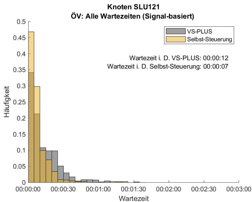
Abbildung 128: Häufigkeitsverteilung der Wartezeiten für den ÖV, mittwochs am Knoten SLU121. In Grau ist die Verteilung des Nullfalles (VS-PLUS) und in Gelb die der Selbst-Steuerung abgebildet.
