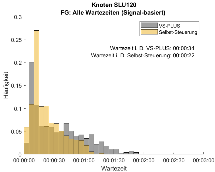
Abbildung 70: Häufigkeitsverteilung der Wartezeiten für den FV, donnerstags am Knoten SLU120. In Grau ist die Verteilung des Nullfalles (VS-PLUS) und in Gelb die der Selbst-Steuerung abgebildet.
