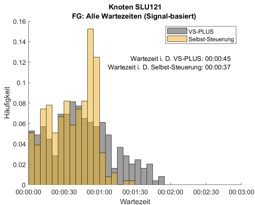
Abbildung 27: Häufigkeitsverteilung der Wartezeiten für den FV in der dienstags Morgenspitze, Knoten SLU121. In Grau ist die Verteilung des Nullfalles (VS-PLUS) und in Gelb die der Selbst-Steuerung abgebildet.
