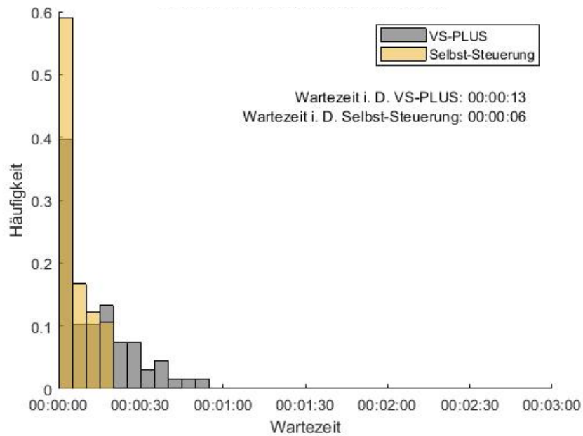
Abbildung 131: : Häufigkeitsverteilung der Wartezeiten für den ÖV am Signalgeber 1 in der Morgenspitze am Knoten SLU121. In Grau ist die Verteilung des Nullfalles (VS-PLUS) und in Gelb die der Selbst-Steuerung abgebildet.
