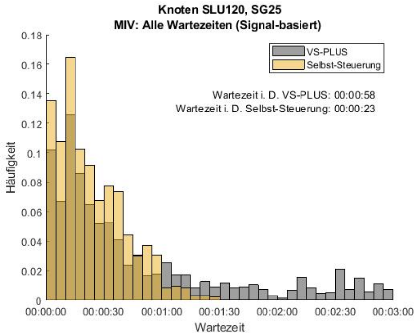
Abbildung 143: Häufigkeitsverteilung der Wartezeiten für den MIV in der dienstags Morgenspitze, Signalgeber 25, Knoten SLU120. In Grau ist die Verteilung des Nullfalles (VS-PLUS) und in Gelb die der Selbst-Steuerung abgebildet.
