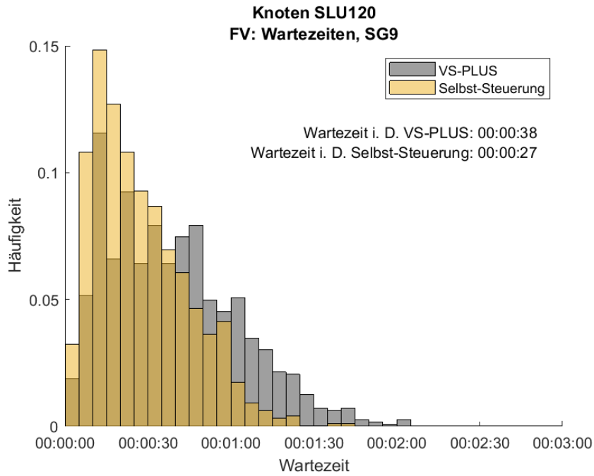
Abbildung 81: Häufigkeitsverteilung der Wartezeiten für den FV am Signalgeber 9 im gesamten Messzeitraum am Knoten SLU120. In Grau ist die Verteilung des Nullfalles (VS-PLUS) und in Gelb die der Selbst-Steuerung abgebildet.
