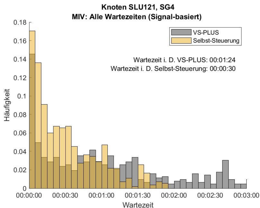
Abbildung 158: Häufigkeitsverteilung der Wartezeiten für den MIV in der dienstags Abendspitze, Signalgeber 4, Knoten SLU121. In Grau ist die Verteilung des Nullfalles (VS-PLUS) und in Gelb die der Selbst-Steuerung abgebildet.
