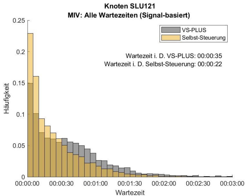
Abbildung 166: Häufigkeitsverteilung der Wartezeiten für den MIV am Freitag, Knoten SLU121. In Grau ist die Verteilung des Nullfalles (VS-PLUS) und in Gelb die der Selbst-Steuerung abgebildet.
