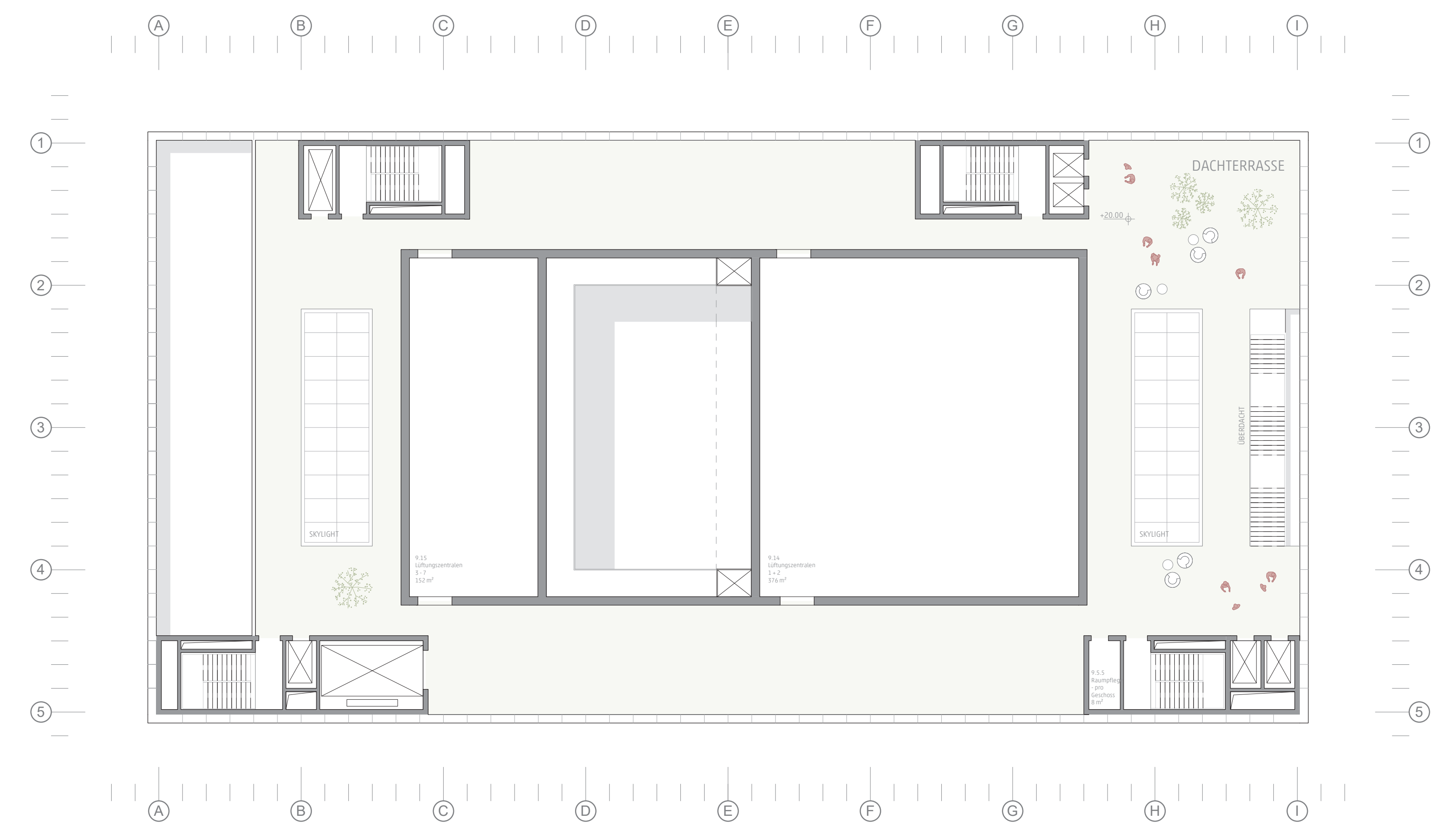
Grundriss DG | 1:200
