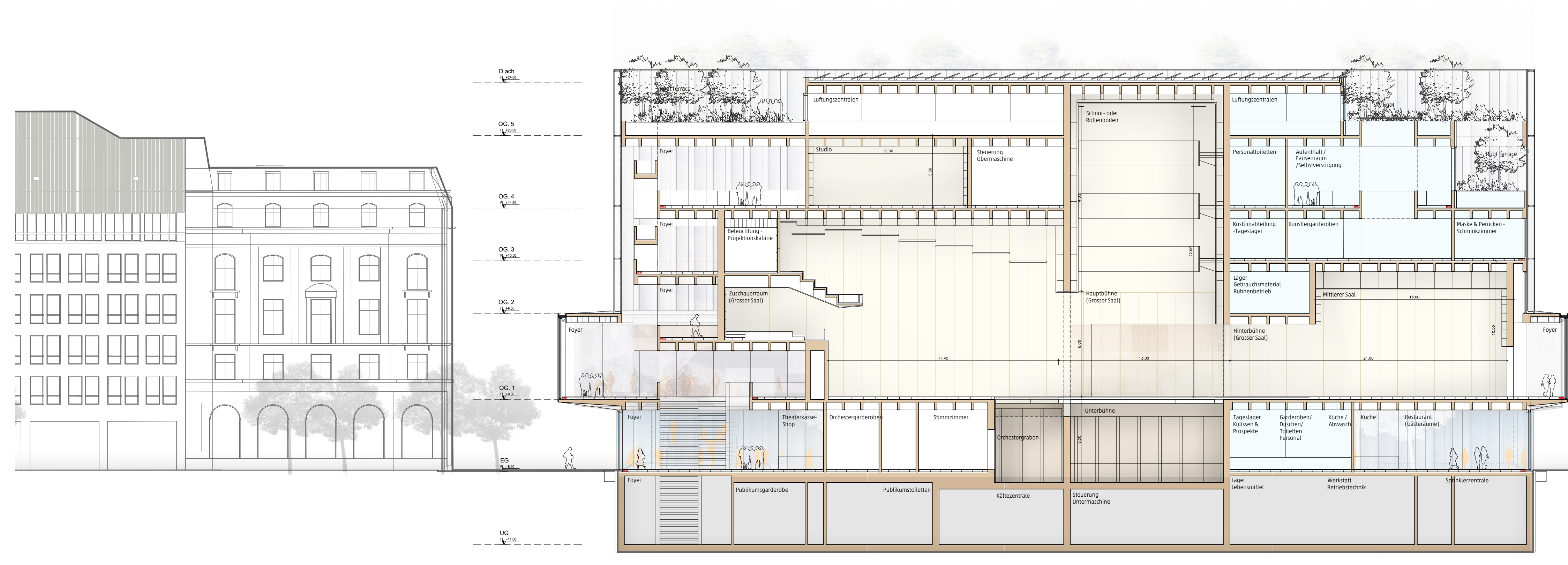
Schnitt F | 1:200
