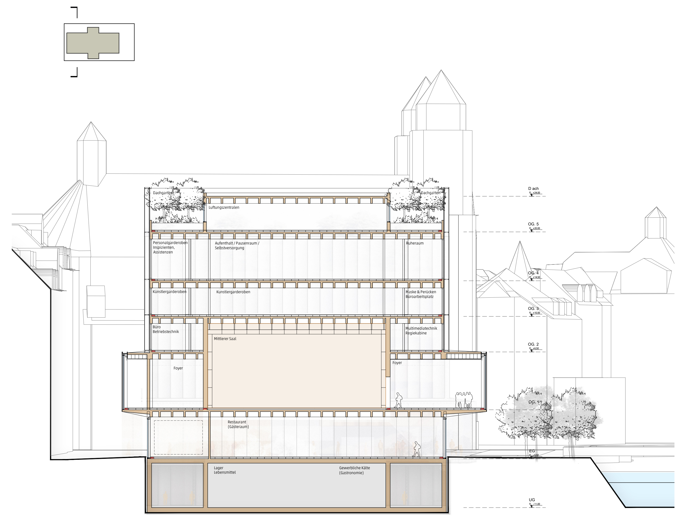
Schnitt D | 1:200
