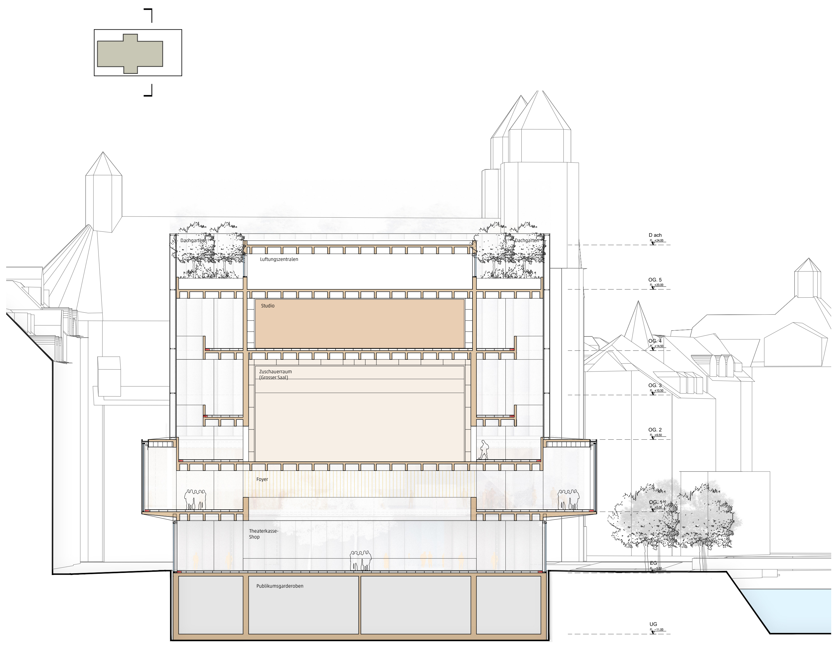
Schnitt B | 1:200
