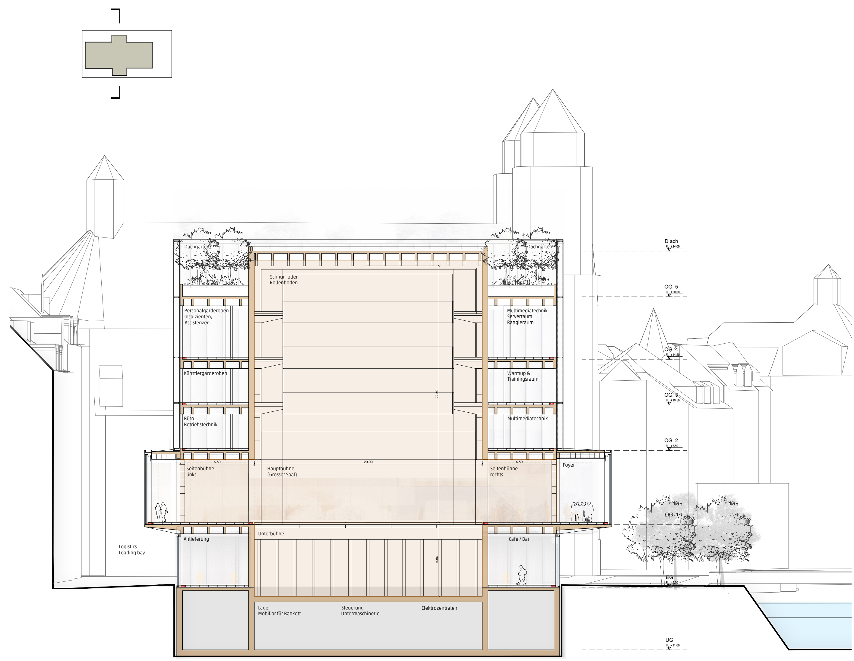
Schnitt C | 1:200
