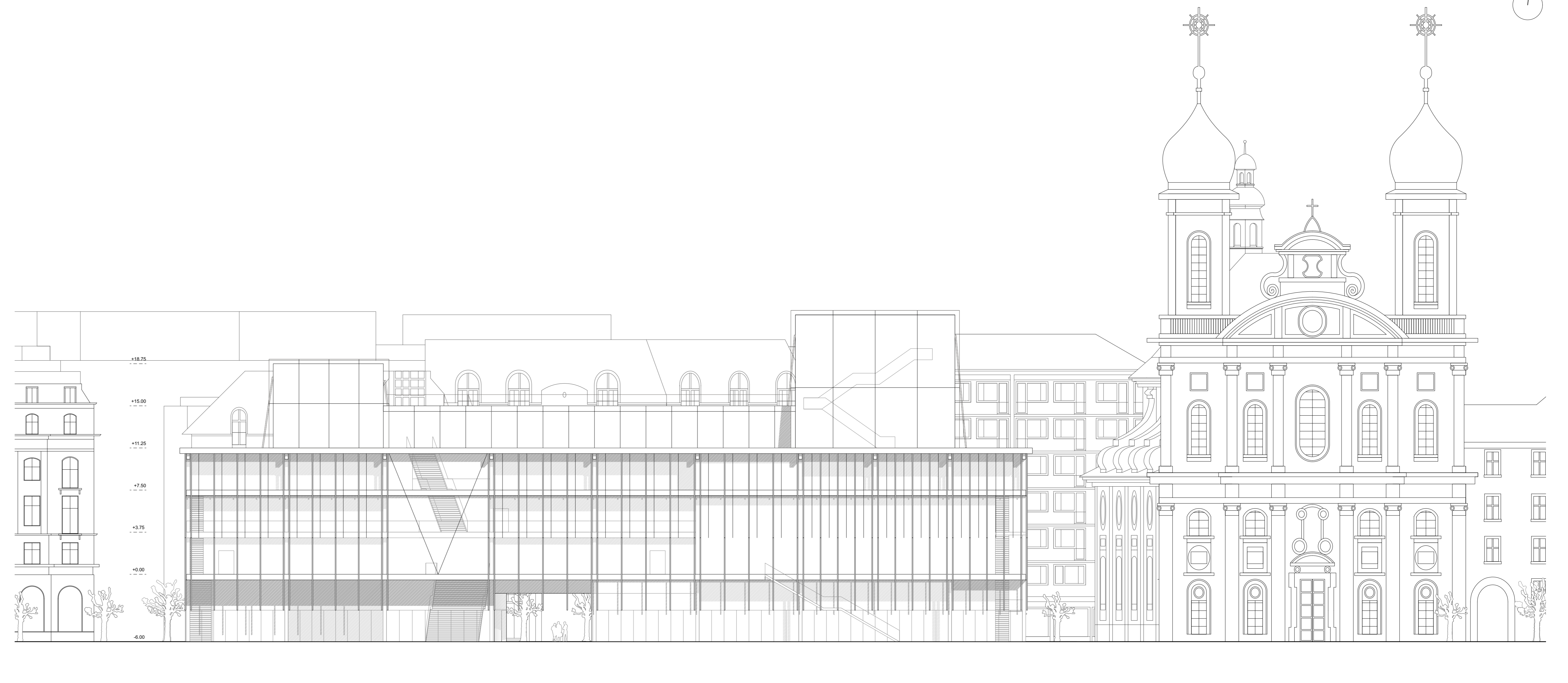
NORDFASSADE 1:200
