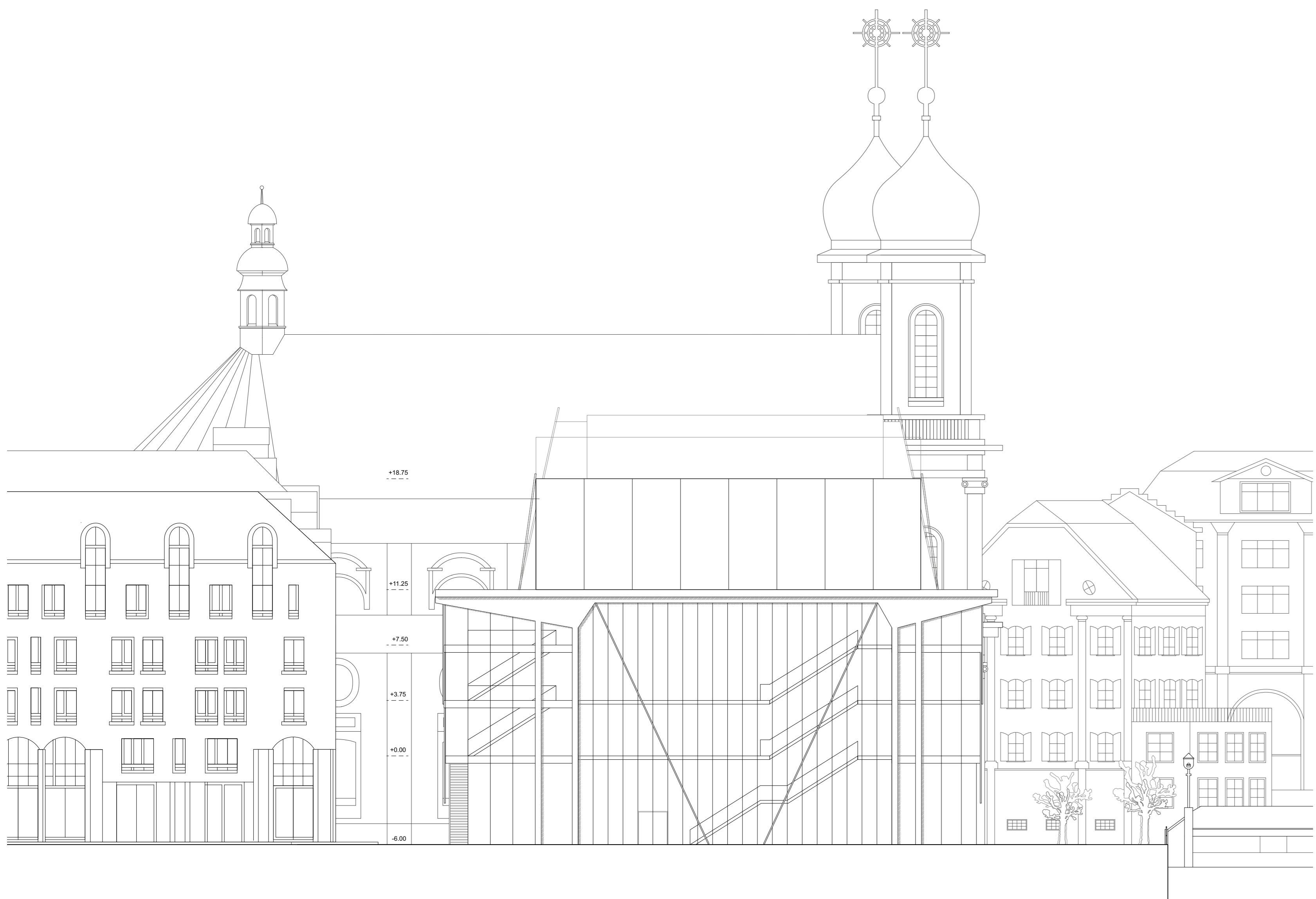
OSTFASSADE 1:200 VORHANG AUF!
